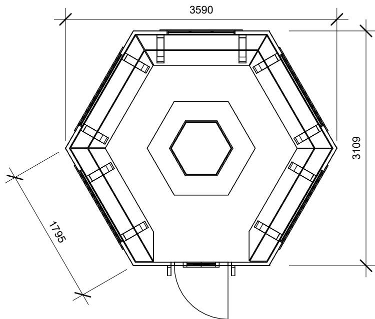
SCHAAL (1:50)
